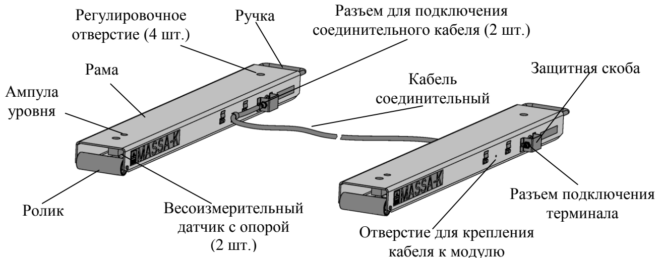
Рисунок 8.1 – Модуль взвешивающий 4D-B_
